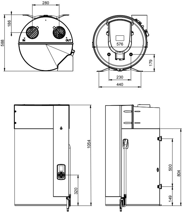
Aéromax VM R290 100
