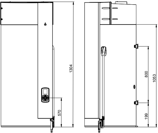
Aéromax VM R290 150
