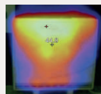
Acumulador de calor Temp. superficial 44,8 °C
