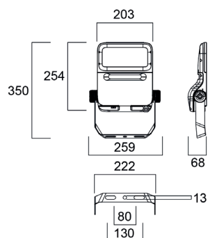
Concord Raiden 3.000 lm
