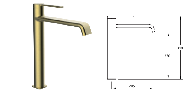
Mezclador alto con aireador y flexibles M-10 3/8" x 500 mm. Tall mixer, aerator, flexible hoses M-10 3/8" x 500 mm. Mitigeur Lavabo bec haut, aérateur, raccords flexibles M-10 3/8" x 500 mm
