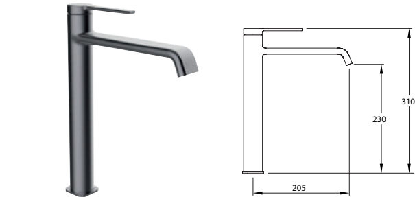
Mezclador alto con aireador y flexibles M-10 3/8" x 500 mm. Tall mixer, aerator, flexible hoses M-10 3/8" x 500 mm. Mitigeur Lavabo bec haut, aérateur, raccords flexibles M-10 3/8" x 500 mm
