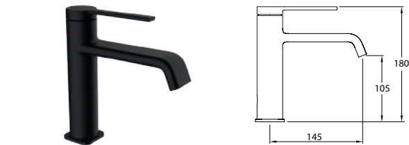
Mezclador con aireador y flexibles M-10 3/8" x 500 mm. Mixer, aerator, flexible hoses M-10 3/8" x 500 mm. Mitigeur lavabo, aérateur, raccords flexibles M-10 3/8" x 500 mm
