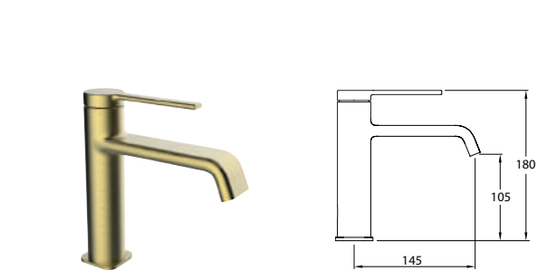
Mezclador con aireador y flexibles M-10 3/8" x 500 mm. Mixer, aerator, flexible hoses M-10 3/8" x 500 mm. Mitigeur lavabo, aérateur, raccords flexibles M-10 3/8" x 500 mm
