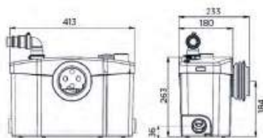
Dimensiones (mm)
