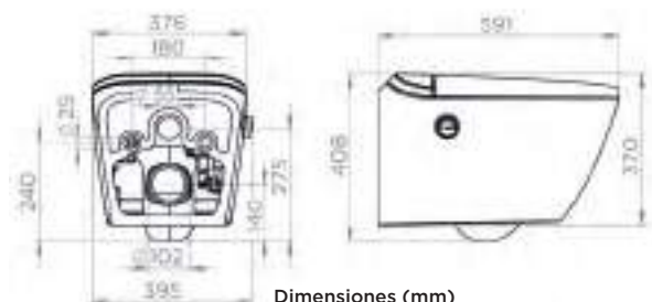
Dimensiones (mm)
