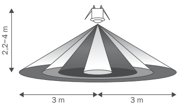
Detector de movimiento
