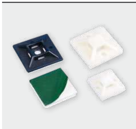
Bases adhesivas Uso interior — Material PA 6.6
