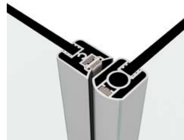
POSICIÓN ABIERTA
