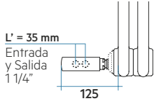
Conexión en Colector (Figura 9)
