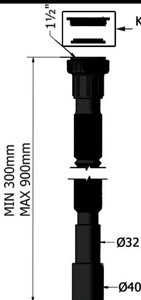
COTAS
